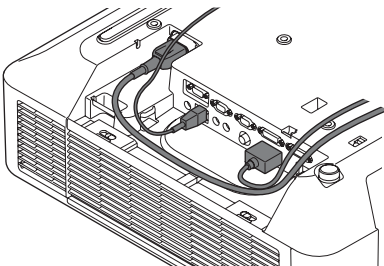
端子盖中的电缆配线示例
