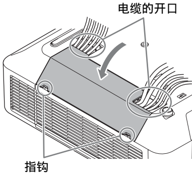
端子盖中的电缆配线示例
